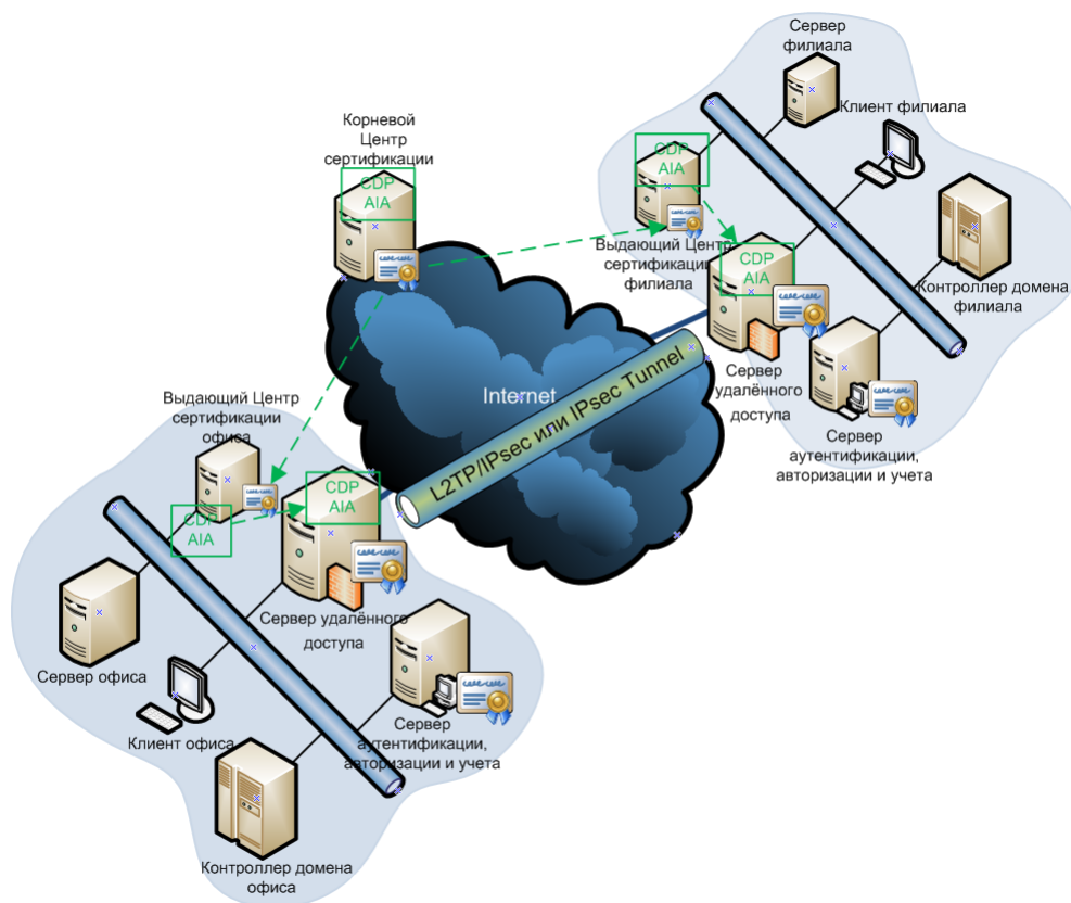
Рисунок 31. Подключение Site-to-Site
