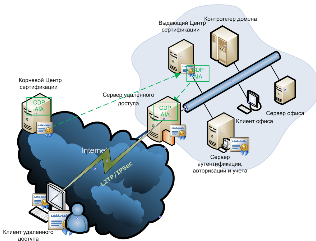
Рисунок 28. Подключение Client-to-Site
