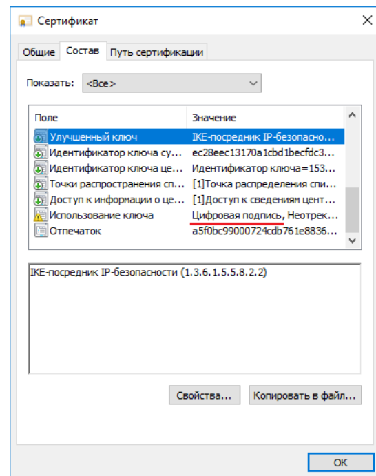
Рисунок 7. Назначение сертификата
