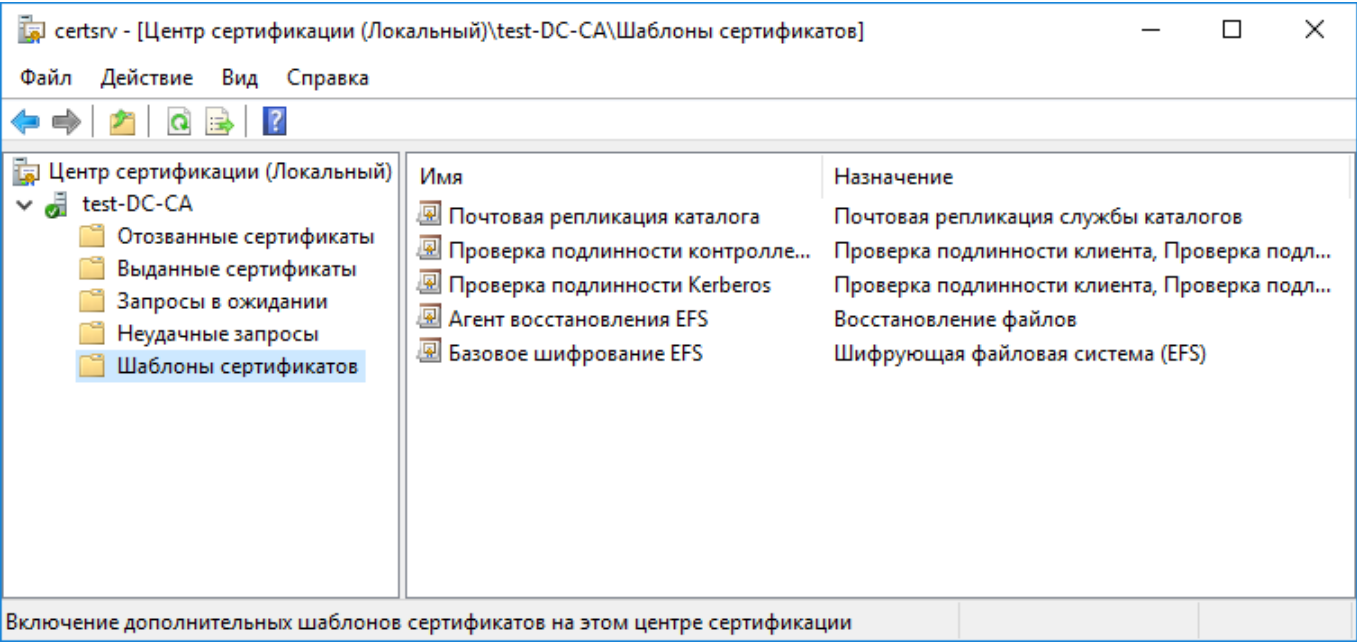
Рисунок 11. Консоль центра сертификации
