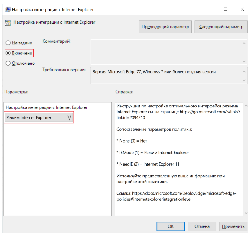
Рисунок 9. Настройка интеграции с Internet Explorer
