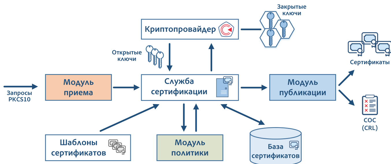
Рисунок 12. Архитектура сервиса сертификации
