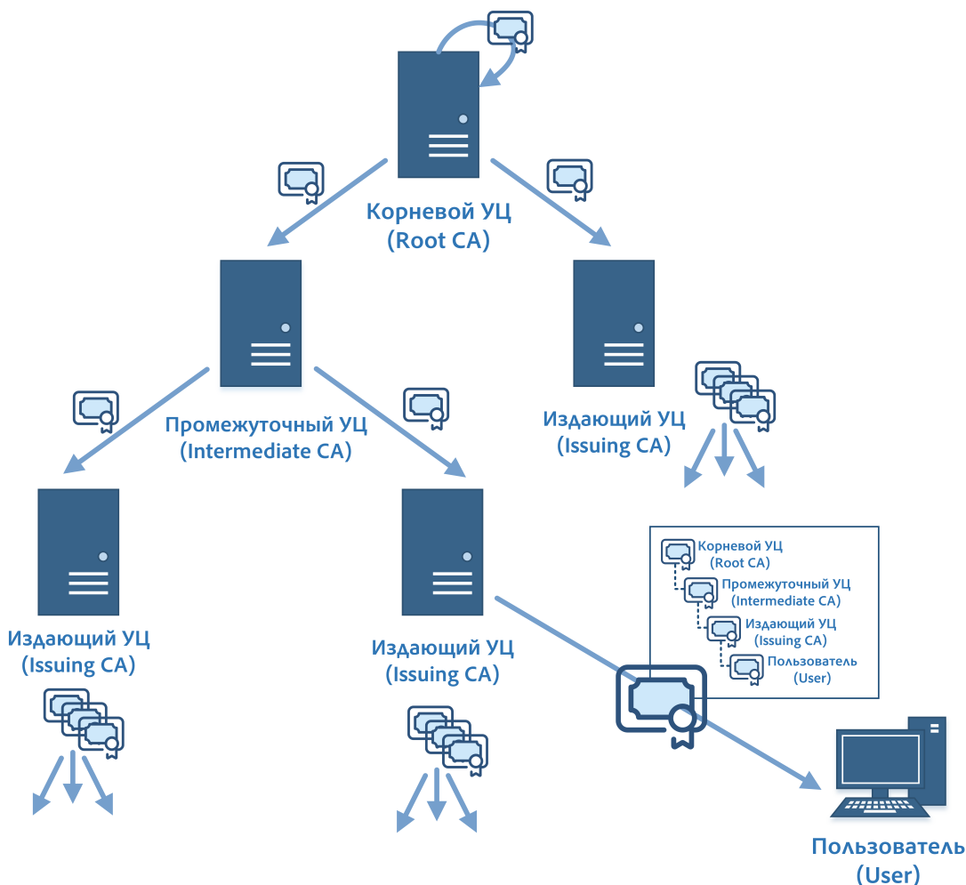
Рисунок 10. Иерархическая модель центров сертификации
